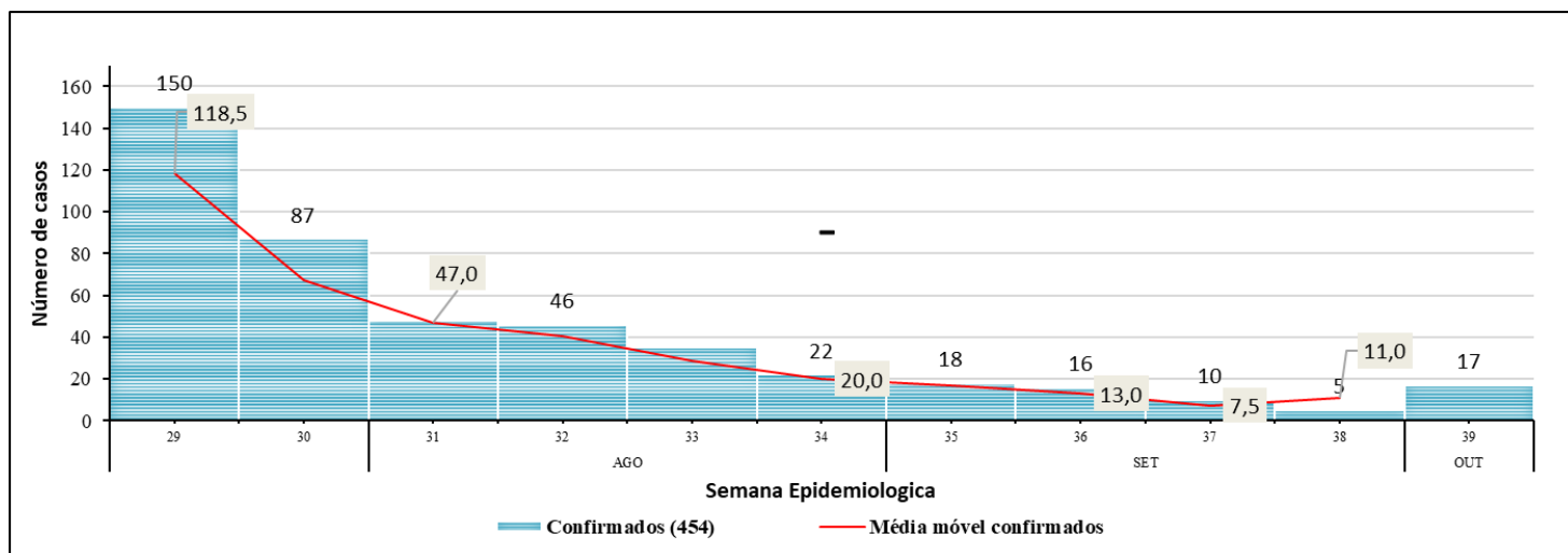
Figura 4. Casos confirmados de Covid-19 e média móvel segundo semana epidemiológica, Cabo Verde, Julho - Outubro, 2022
